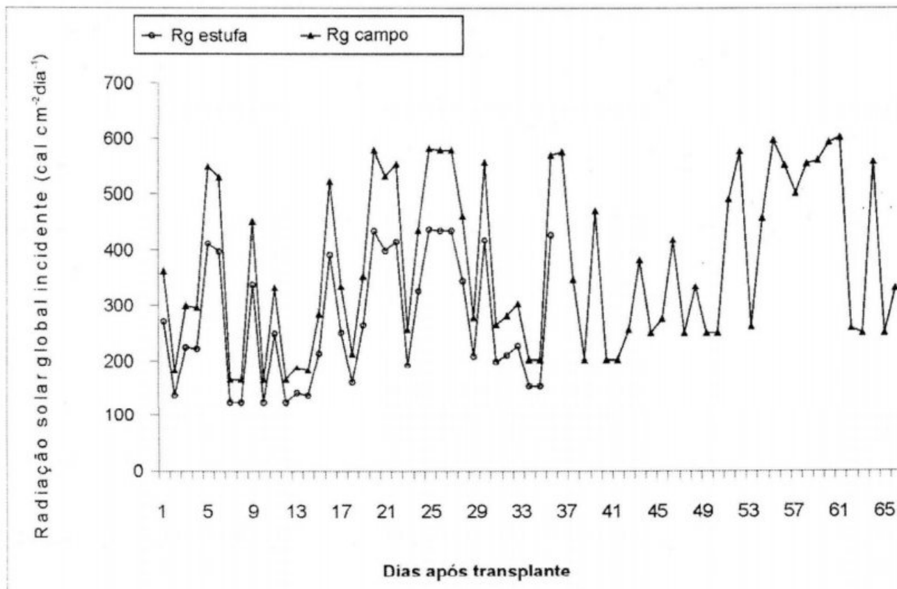
FIGURA 2 - Radiação solar global incidente ( cal\ cm^{-2}\ dia^{-1} ) no interior da estufa e a campo nos períodos de outubro a dezembro de 2002. Universidade Federal de Santa Maria, RS, 2002.
