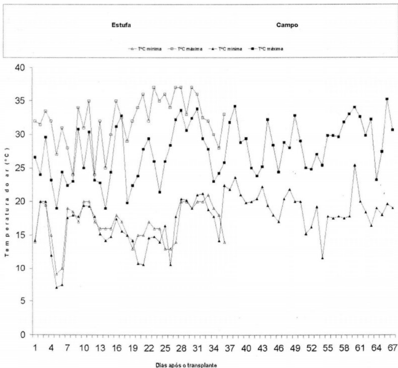
FIGURA 1 - Temperatura do ar (°C) no interior da estufa e a campo nos períodos de outubro a dezembro de 2002. Universidade Federal de Santa Maria, RS. 2002.
